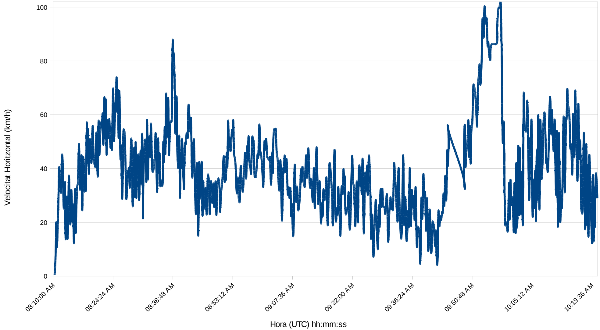
Gràfic Velocitat Horizontal - Temps (UTC) durant el vol
