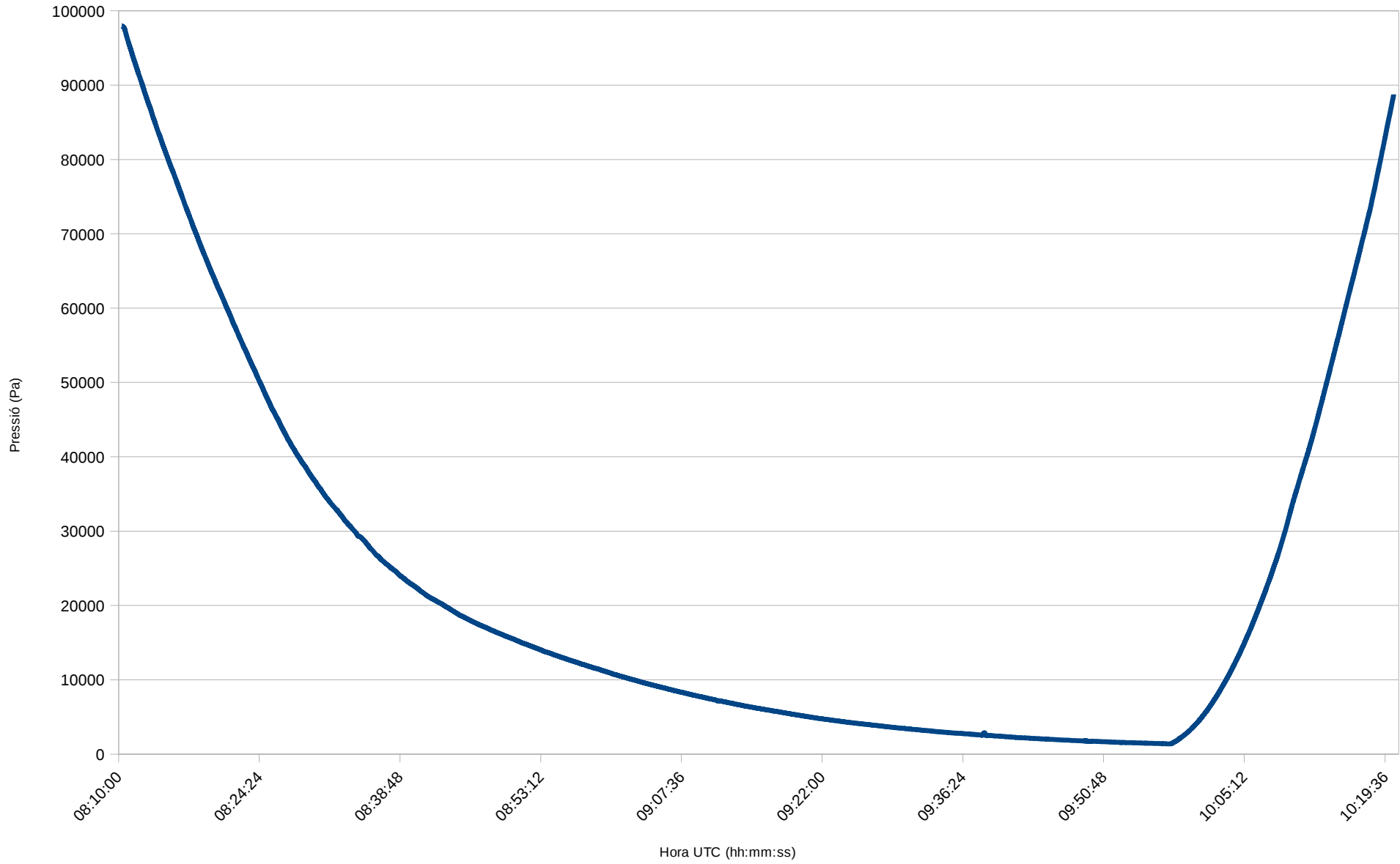
Gràfic Pressió - Temps (UTC) al llarg de tot el vol
