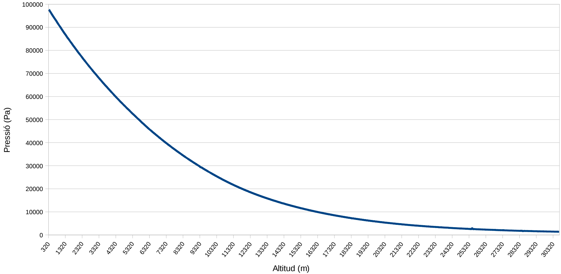
Gràfic de pressió - altitud durant l'ascens
