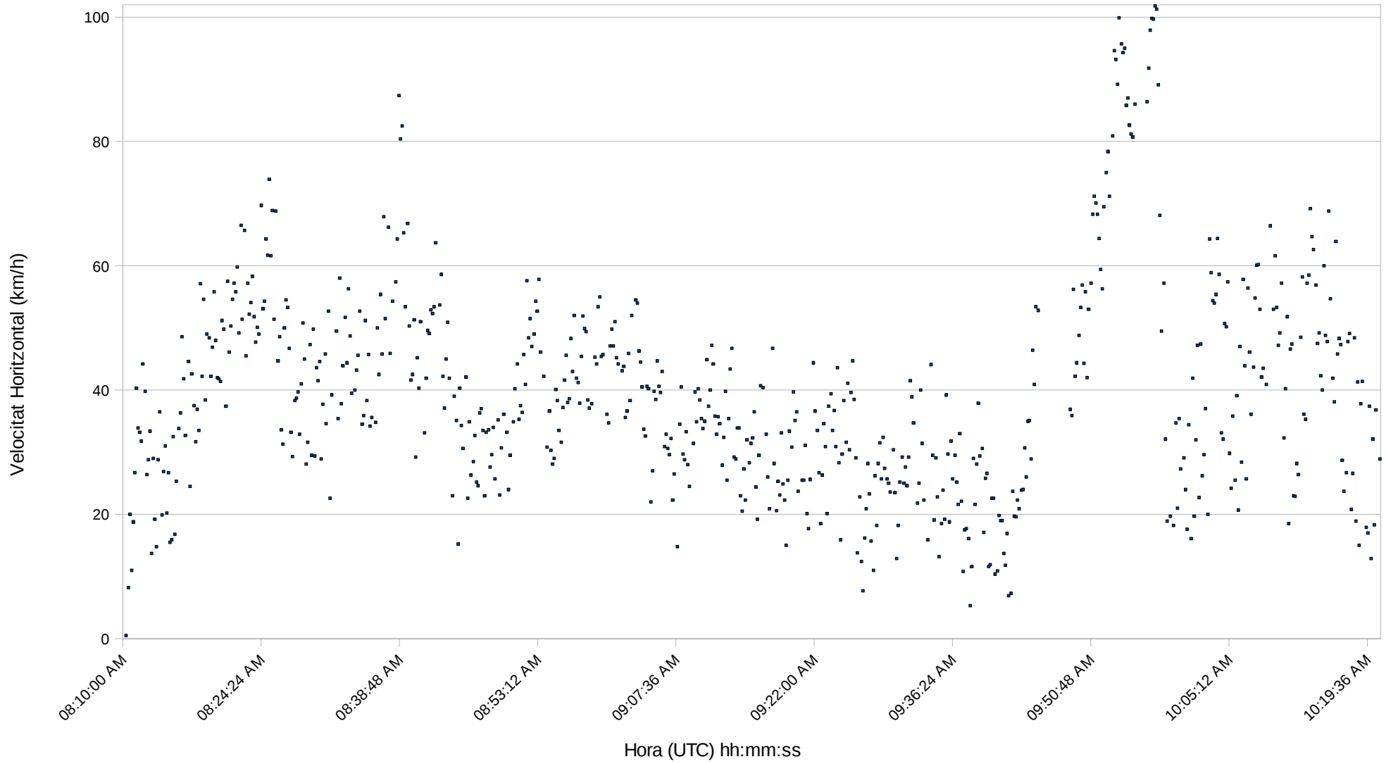
Gràfic Velocitat Horitzontal - Temps (UTC) durant el vol
