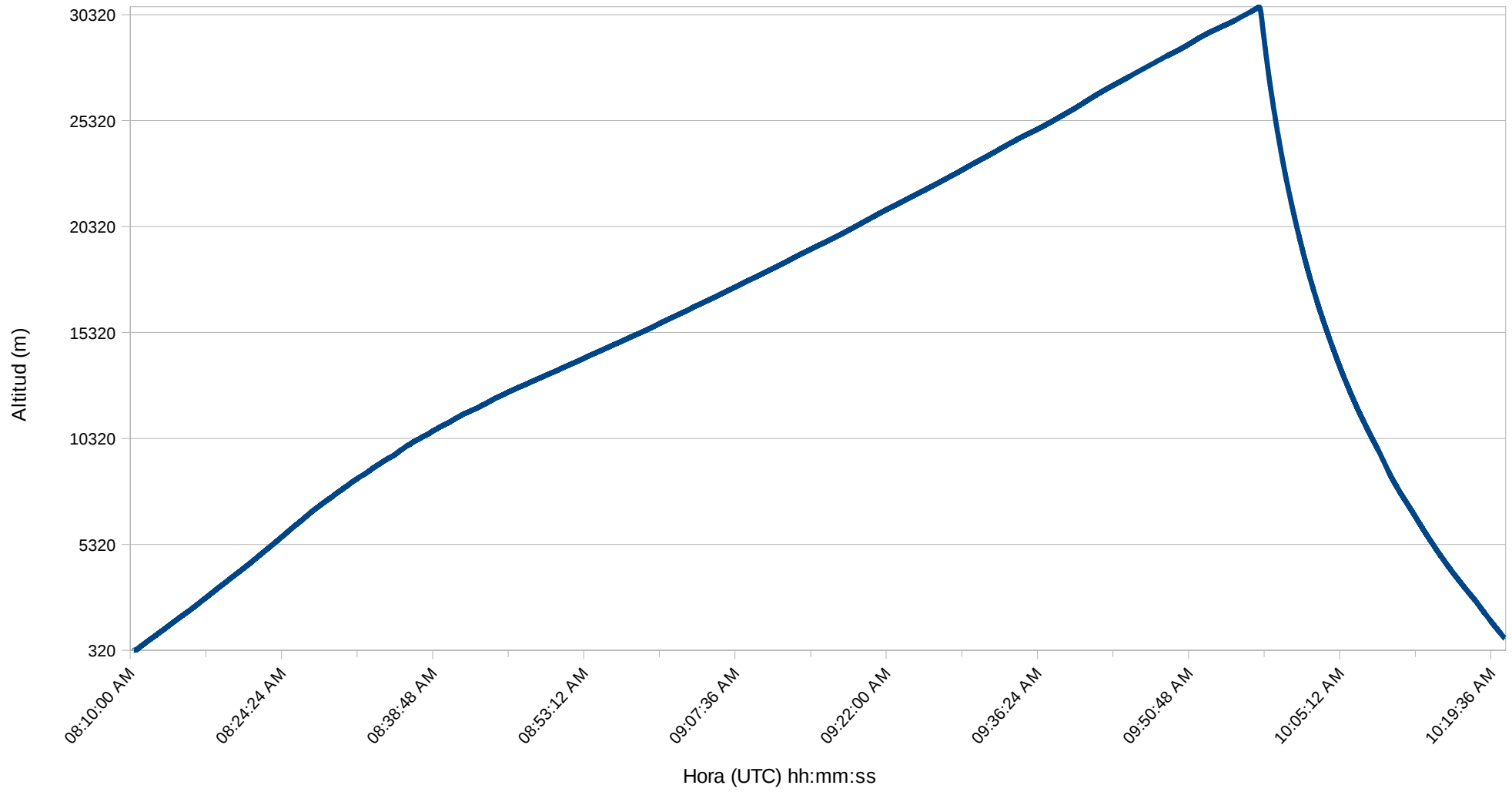
Gràfic de l'altitud - temps (UTC) durant el vol
