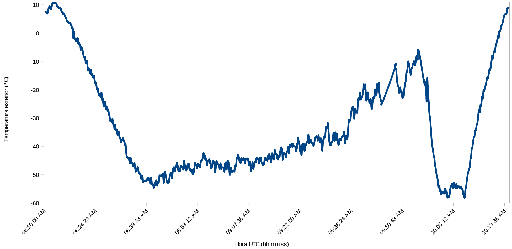
Gràfic temperatura ext. - temps (UTC) durant el vol
