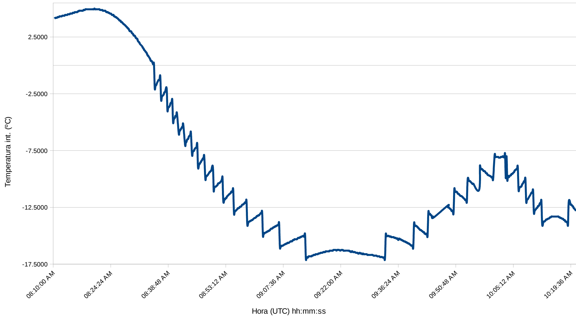
Gràfic temperatura interior - temps (UTC) durant el vol
