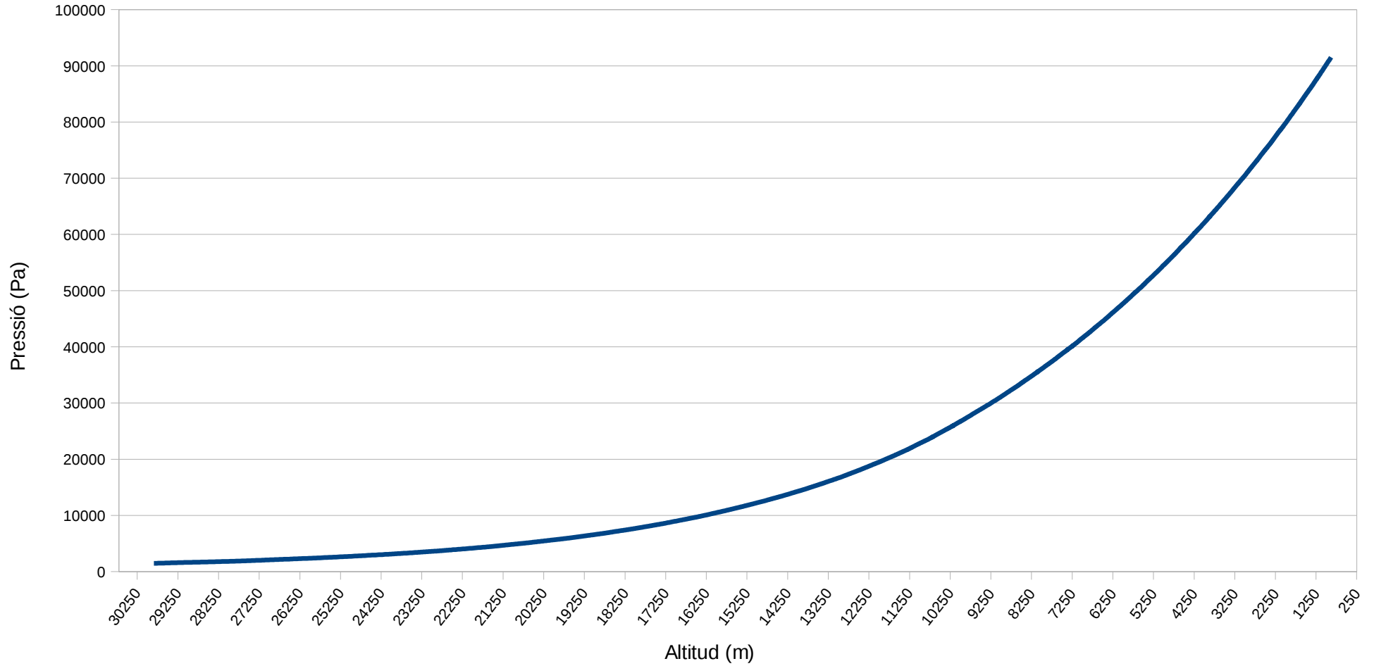
Gràfic de pressió - altitud durant el descens
