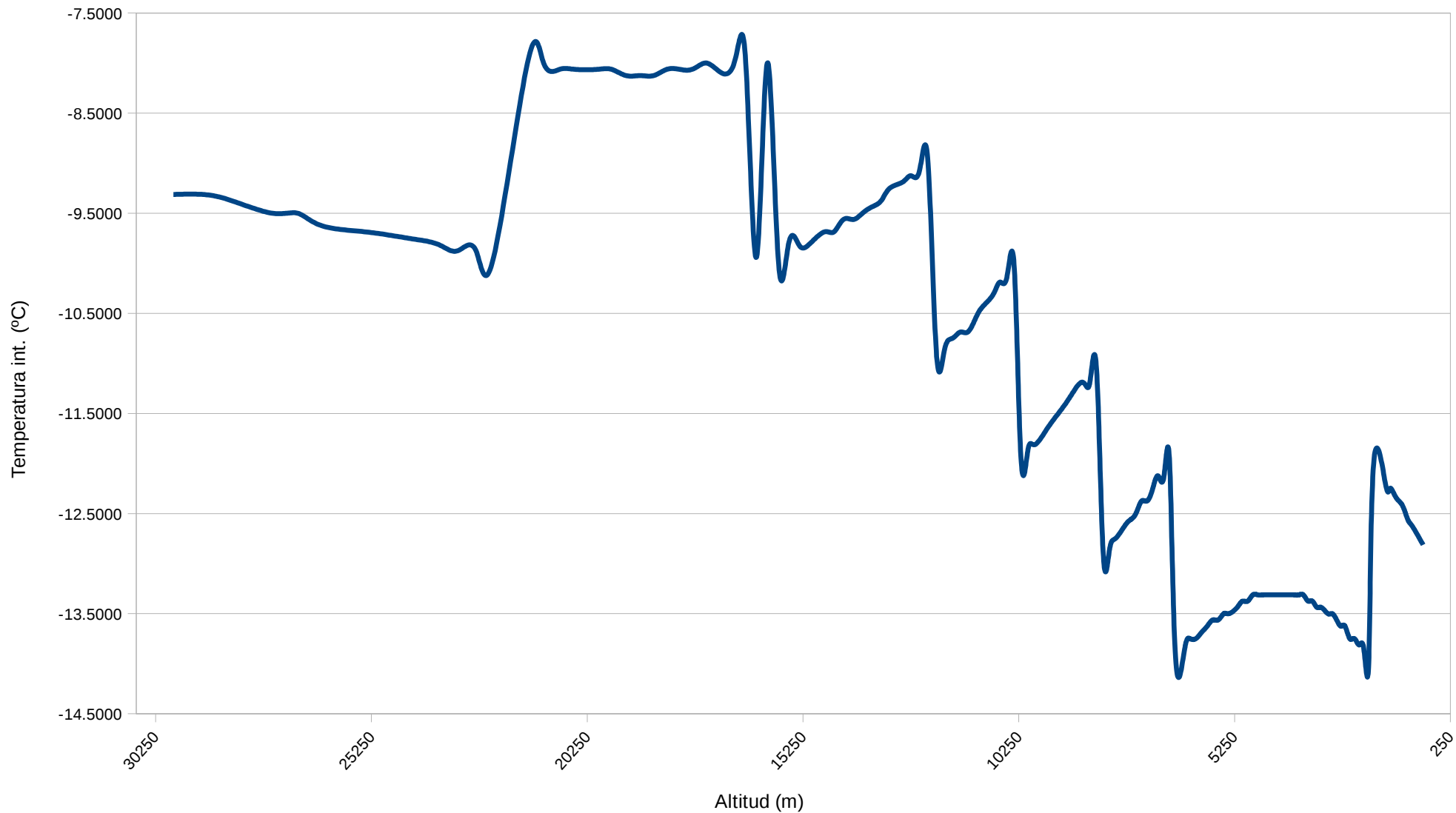
Gràfic Temperatura interna - altitud durant el descens
