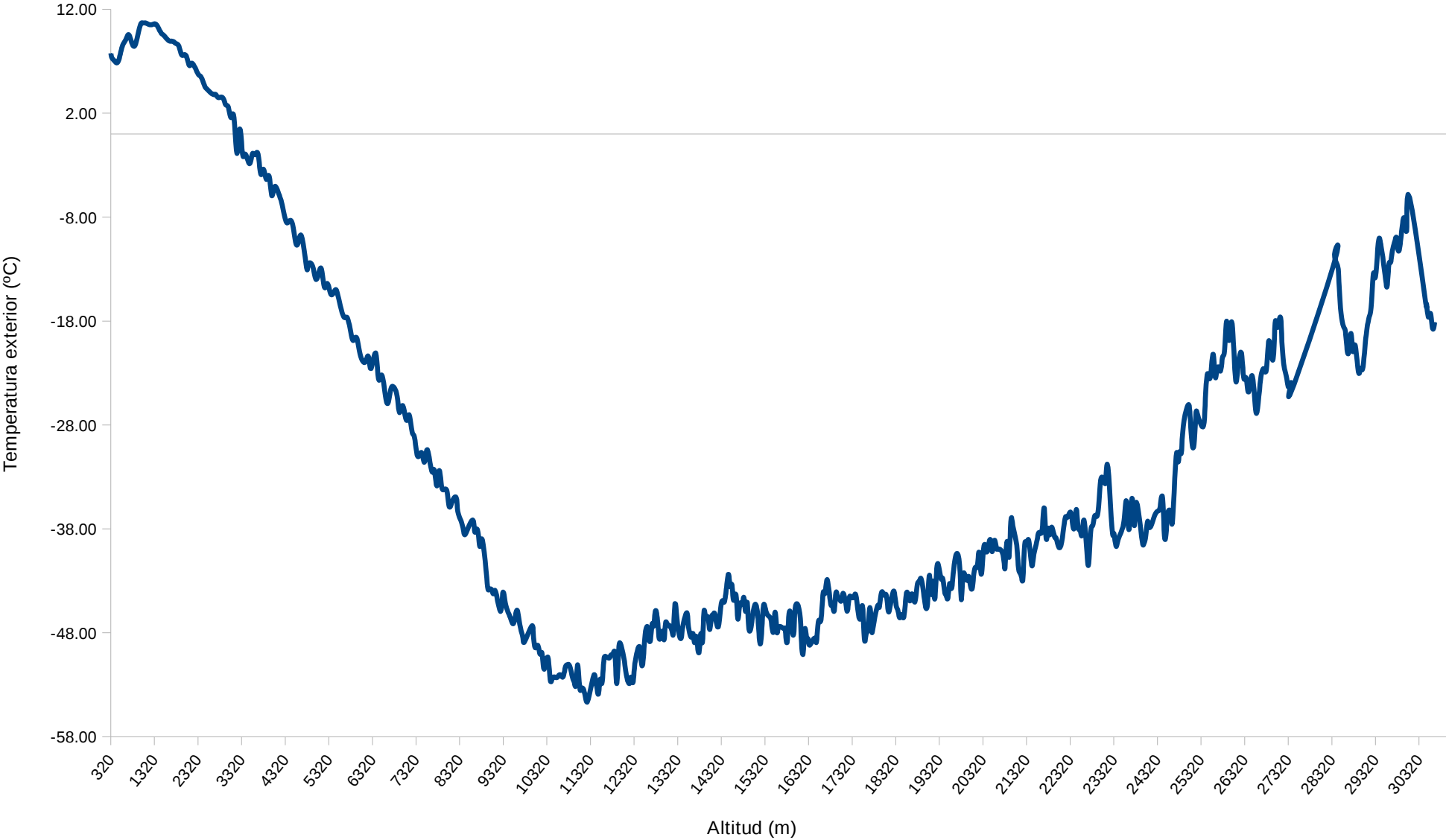
Gràfic temperatura ext - altitud durant l'ascens
