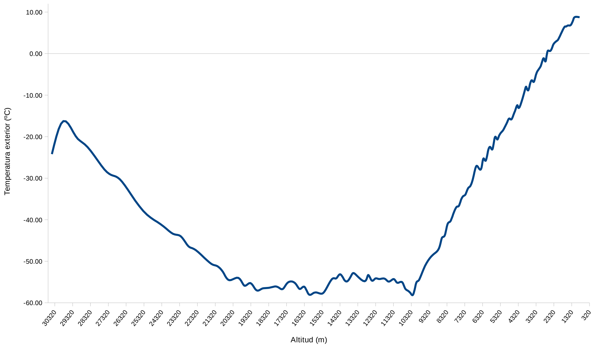
Gràfic temperatura ext - altitud durant el descens
