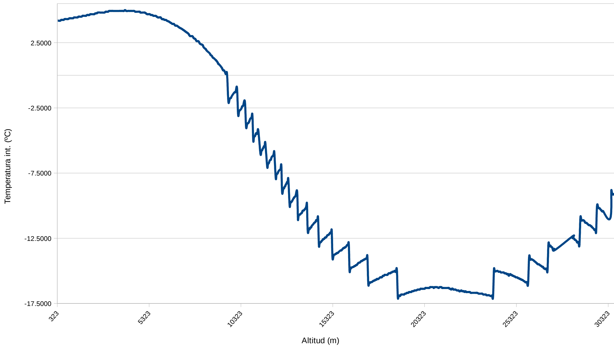
Gràfic Temperatura interna - altitud durant l'ascens
