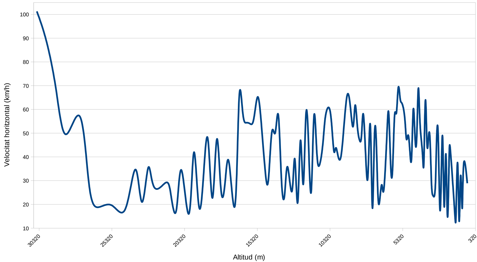
Gràfic velocitat horitzontal - altitud durant el descens
